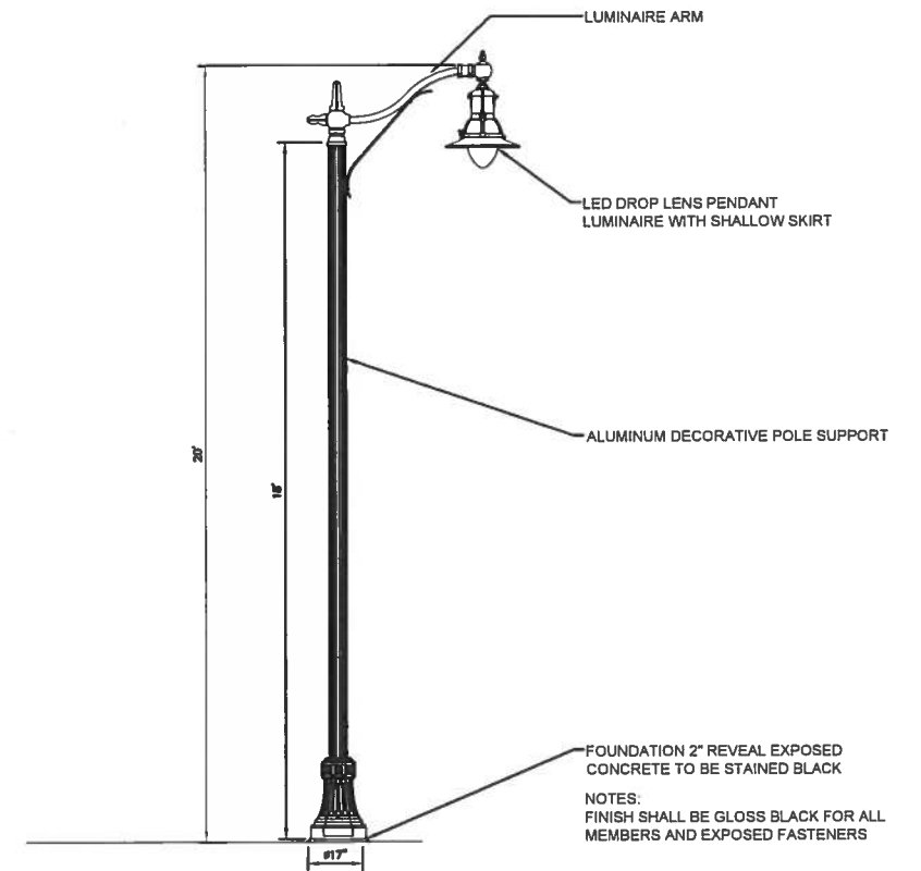
LIGHTPOLE AND LUMINAIRE TYPE (D) RESIDENTIAL
